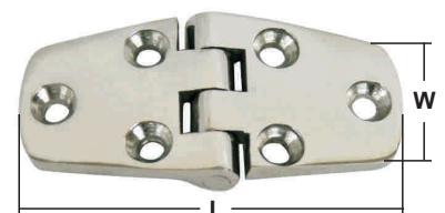
DOOR HINGE precision casted AISI 316
